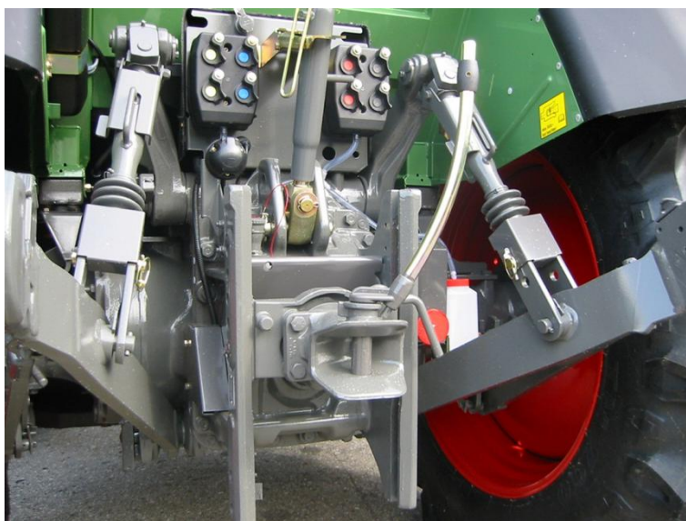
Abbildung 3: Höhenverstellbare nichtselbsttätige Anhängerkupplung mit verlängertem Griff des Kupplungsbolzens (Foto: AGCO-Fendt)
