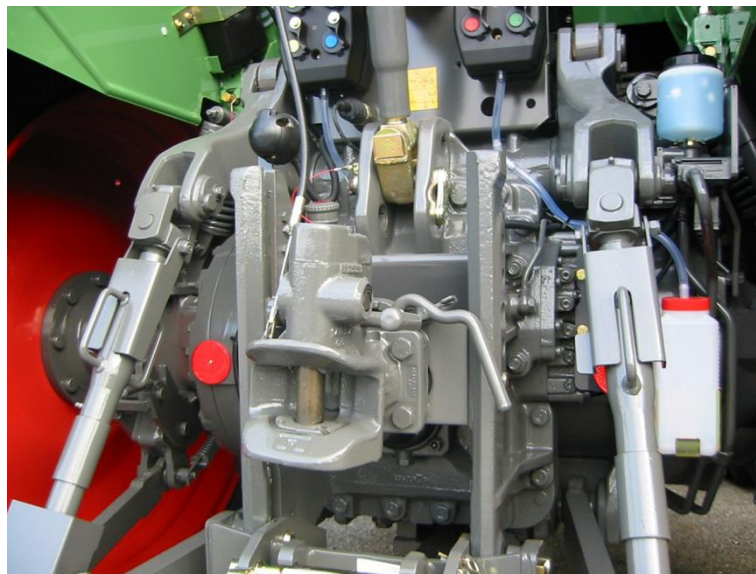
Abbildung 5: Heck eines Standardtraktors mit höhenverstellbarer selbsttätiger Bolzenkupplung mit „Fernbedienung“ vom Traktorsitz (Foto: AGCO-Fendt)
