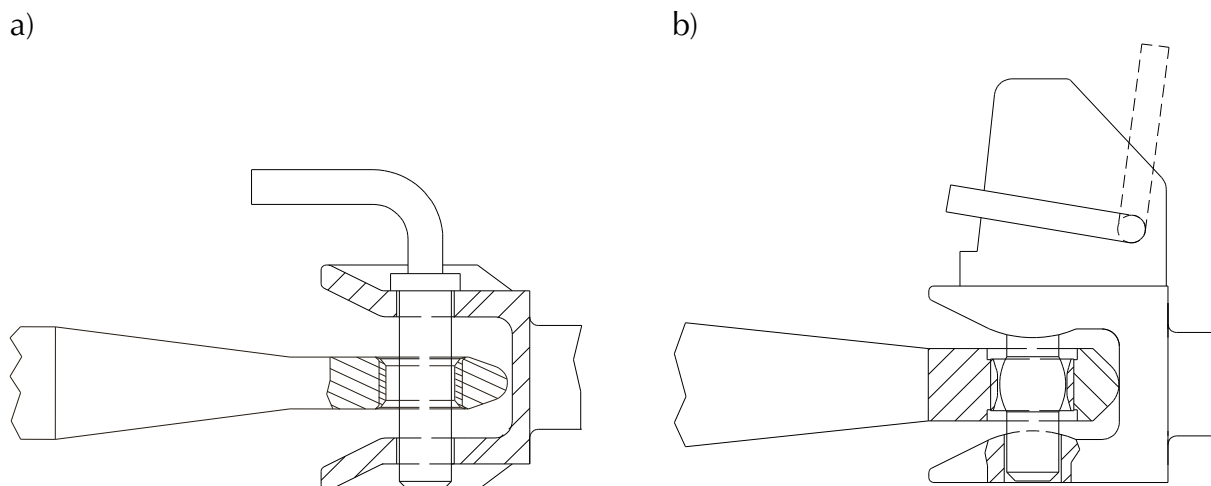
Abbildung 4: Prinzipskizzen von Anhängerkupplungen nach ISO 6489-2, DIN 11028
