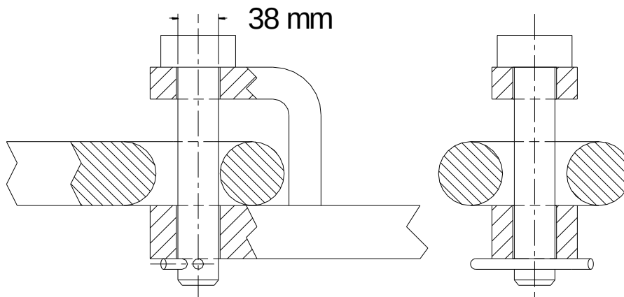
Abbildung 12: Zugpendelanhängung von landwirtschaftlichen Geräten
