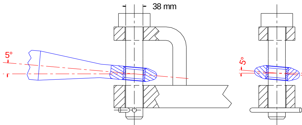
Abbildung A8: Probleme bei Verbindung Zugpendel mit „Hitch“-Zugöse nach ISO 5692-1 und Zugöse 40 nach ISO 8755
