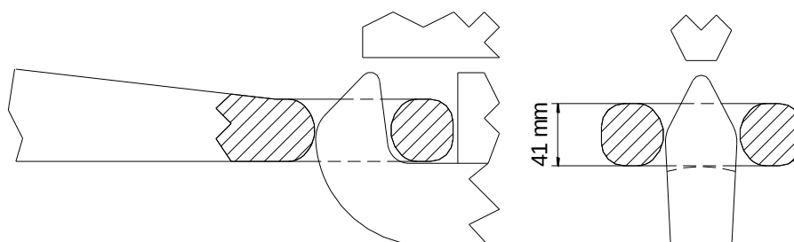
Abbildung 7c: Prinzipskizze des Hitchhakens nach ISO 6489-1 mit Zugöse nach ISO 20019
