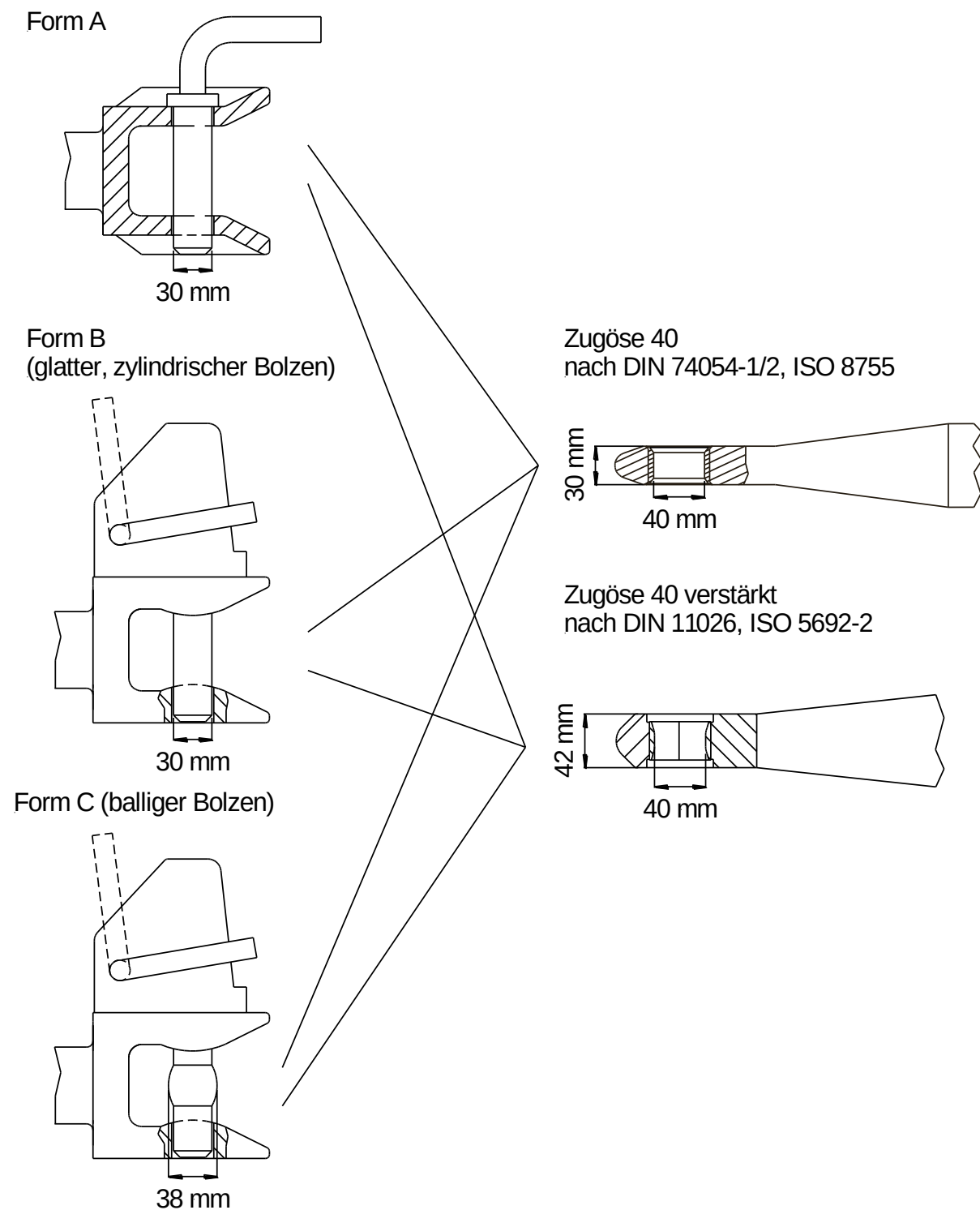
Abbildung A1: Mögliche Kombinationen von Bolzenkupplungen und Zugösen
